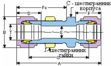
Шестигранник гайки
